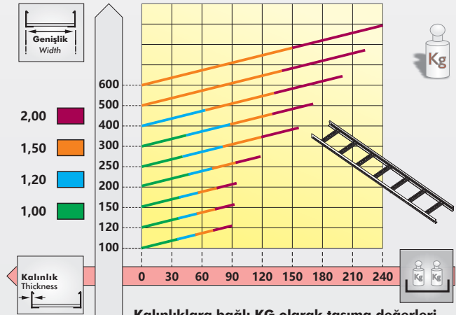
Kalınlıklara bağlı KG olarak taşıma değerleri Carriage values in KG depending on thickness
