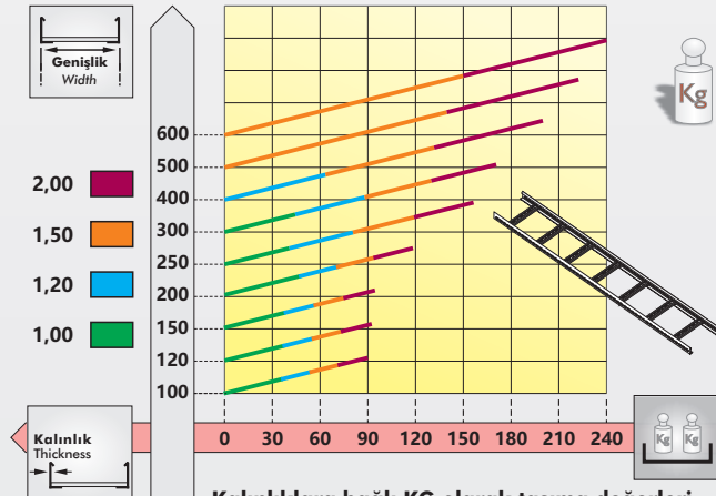
Kalınlıklara baęlı KG olarak taşıma deęerleri Carriage values in KG depending on thickness
