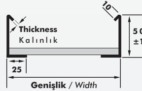
Merdiven Yan Kenar Ölçüleri Dimensions for Side of Ladder Bend
