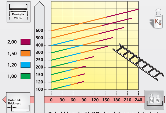
Kalınlıklara baęlı KG olarak taşıma deęerleri Carriage values in KG depending on thickness
