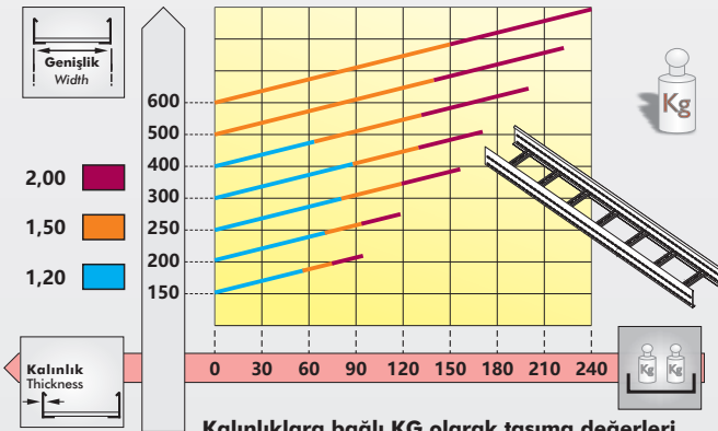
Kalınlıklara bağlı KG olarak taşıma değerleri Carriage values in KG depending on thickness
