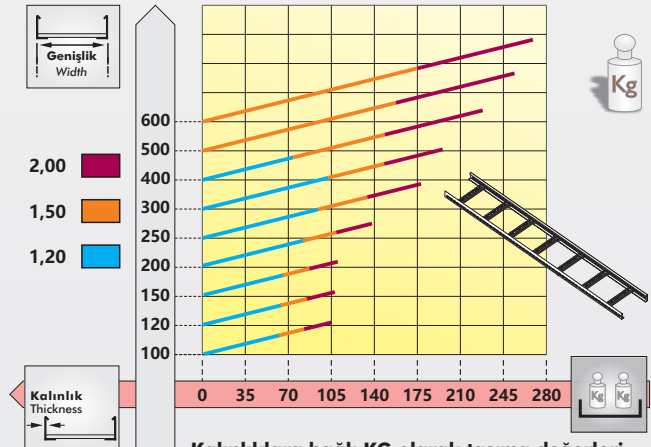
Kalınlıklara bağlı KG olarak taşıma değerleri Carriage values in KG depending on thickness
